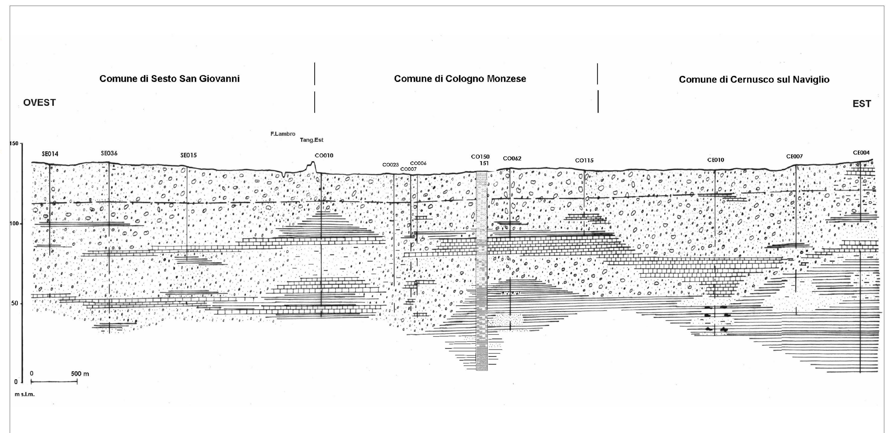
SEZIONE EST-OVEST
