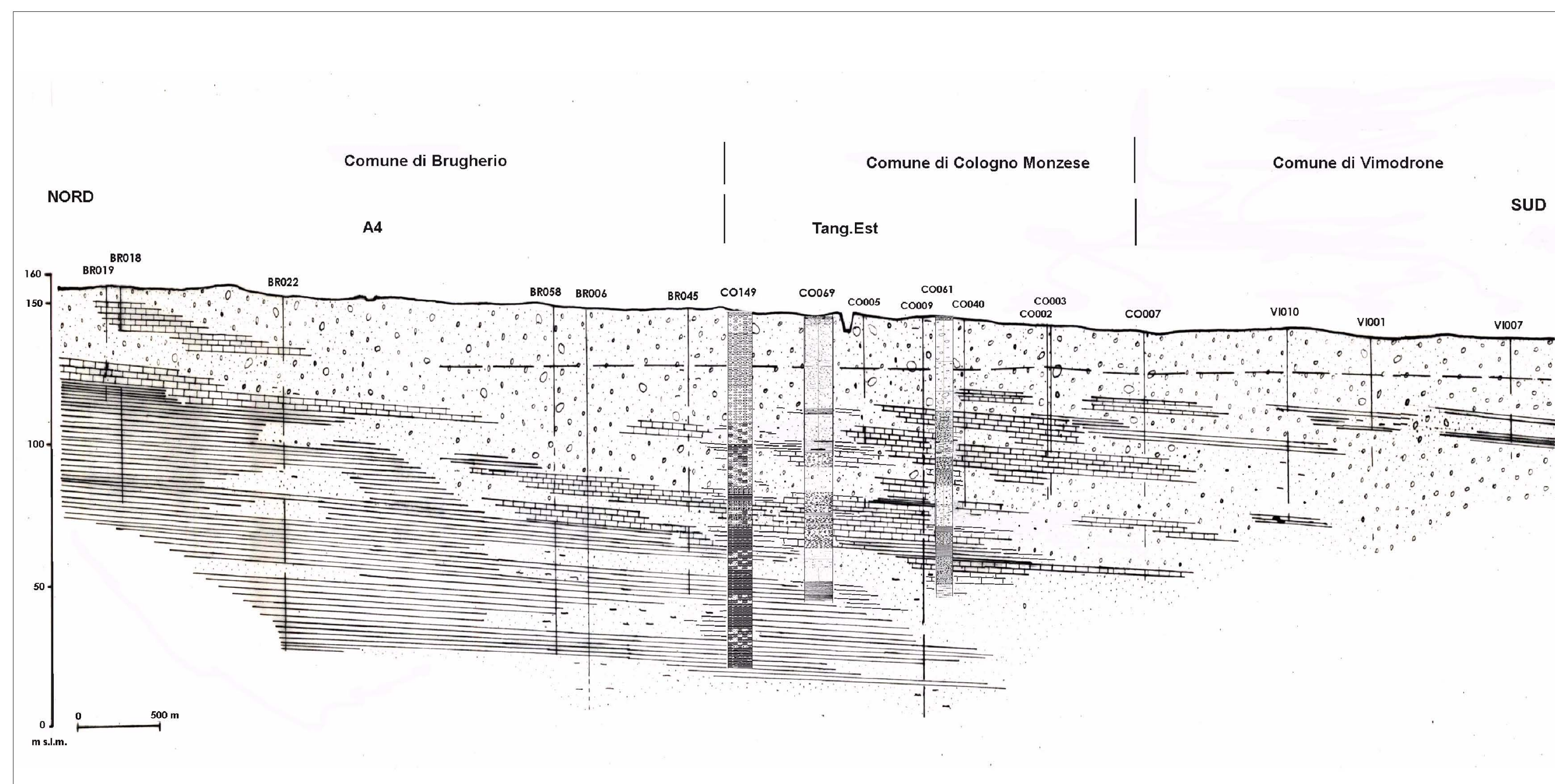
SEZIONE NORD-SUD
